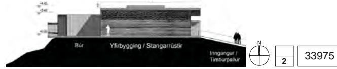
Vesturhlið
