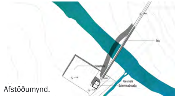
Afstöðumynd. Skipulag Stangarhólsins
